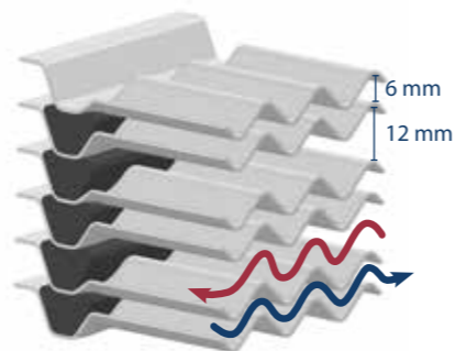
Asymmetrisk High og Low plade princip
