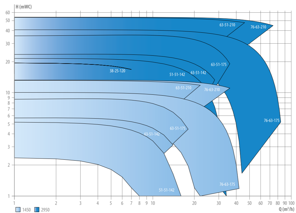
Ydelseskurve - DanPumps S-FP serien - 50 Hz med max. og min. pumpehjuls diameter
